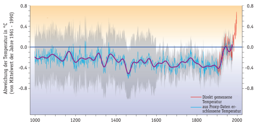
Schwankung der Temperatur der Erdoberfläche in den letzten 1000 Jahren
