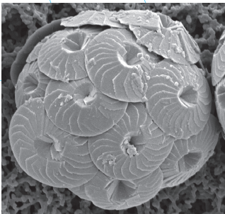
Bei momentaner CO 2 -Konzentration
