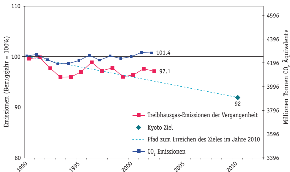
Treibhausgas-Emissionen Europas (EU-15) im Vergleich zur Kyoto-Zielvorgabe
