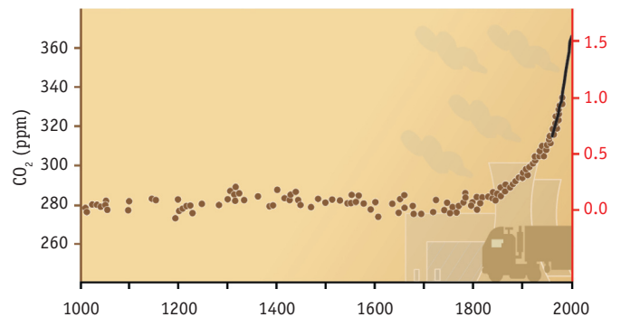
Schwankung der atmosphärischen \text{CO}_2 -Konzentration in den letzten 1000 Jahren
